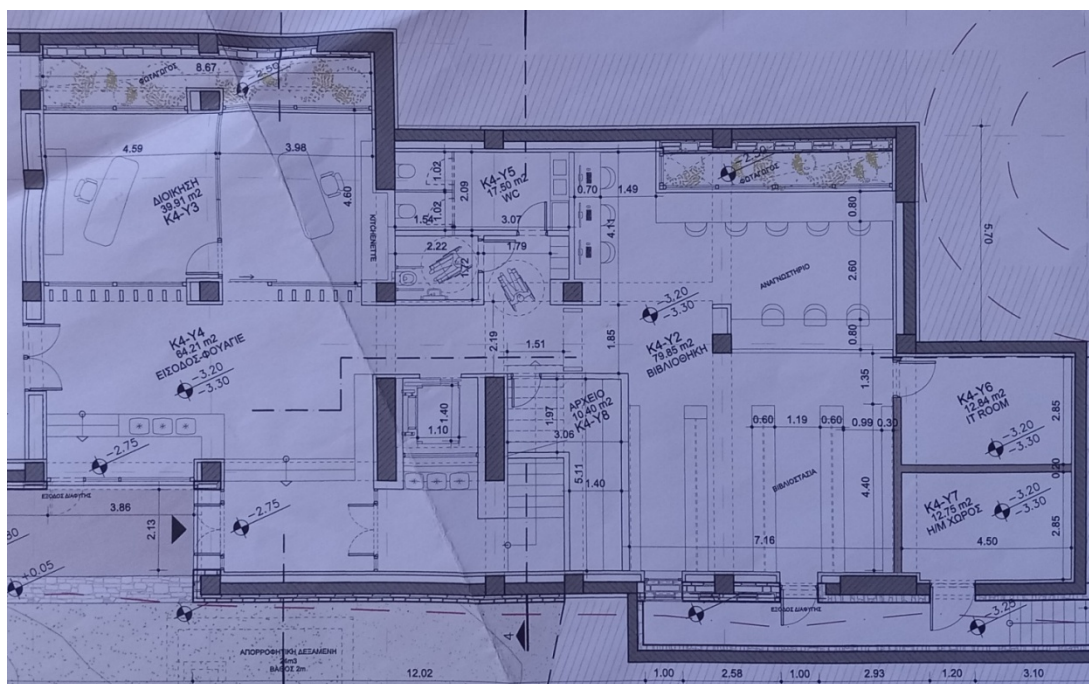
Εικ. 1: Κάτοψη του χώρου Κ4-Υ2 «Βιβλιοθήκη», από την Προμελέτη των νέων κτιρίων του ΠΕΣΚΤΠΤ. Επίσης φαίνεται η σχέση της Βιβλιοθήκης με τον χώρο διοίκησης και άλλους χώρους αμεσης γειτνίασης (όπως πχ ο χώρος Κ4-Υ6 «IT ROOM»).
